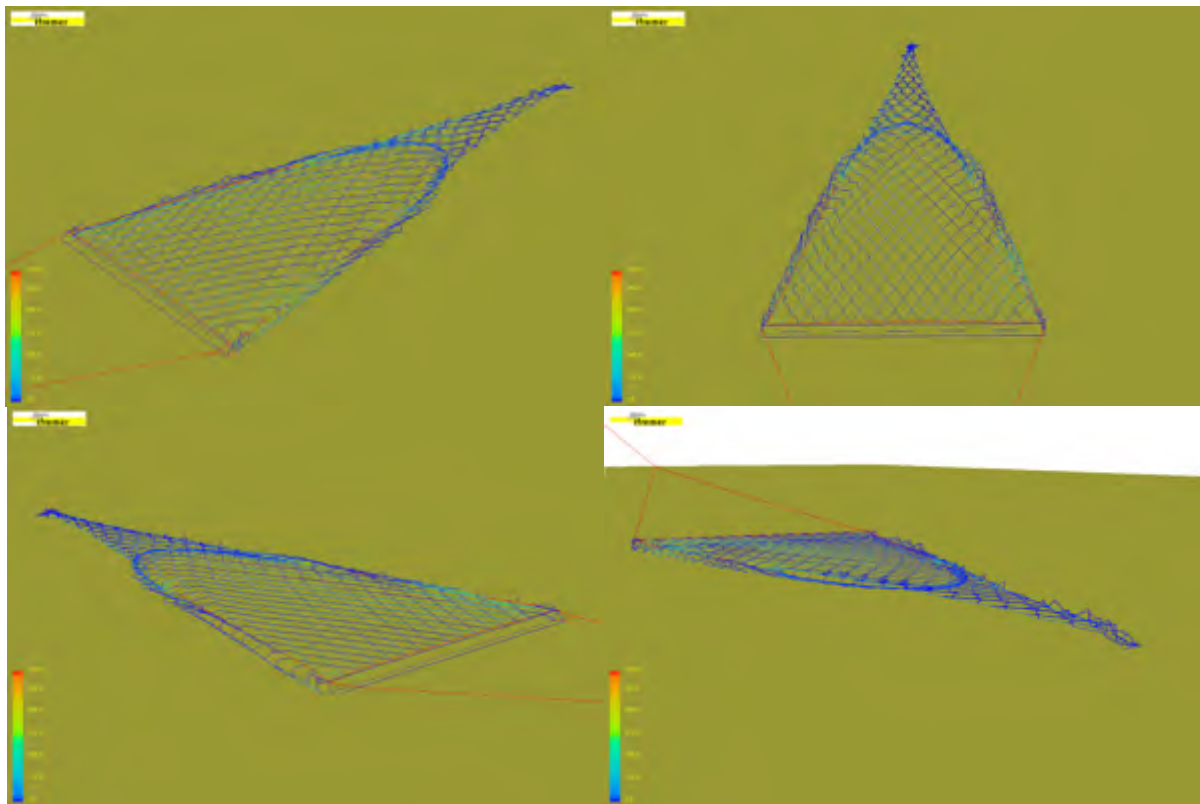
Figuur 4-11: DynamiT simulatie van het orginele boomkornet van de FD-281
