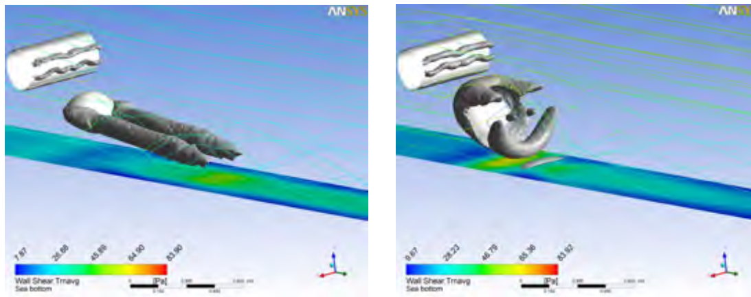
Figuur 4-6: Invloed van de instelhoek op wervelvorming aan de boom met bolkap (DELTARES)
