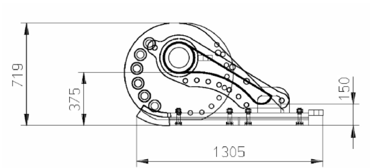
Figuur 3-9: Tweede versie HydroRig ontwerp VCU-TCD juli 2008 – zijaanzicht
