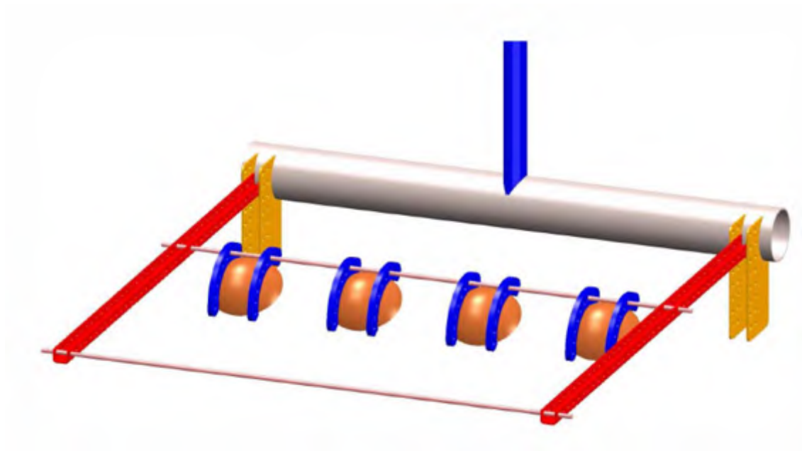
Figuur 3-2: Opstelling model 1:1 in de water-grond goot van DELTARES
