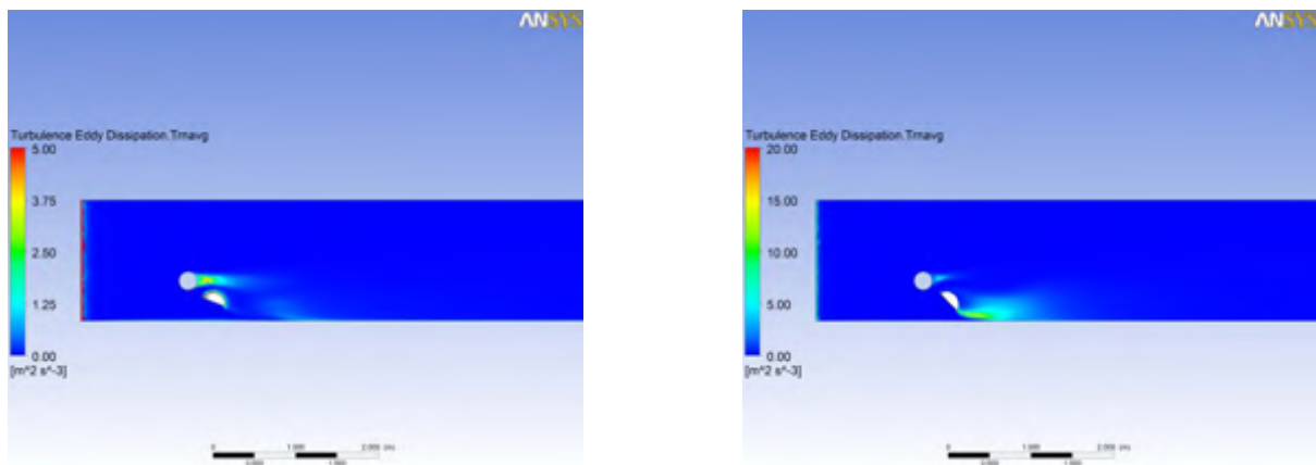
Figuur 4-7: Invloed van de instelhoek op turbulentie aan de boom met bolkap (DELTARES), links 20^\circ en rechts 45^\circ
